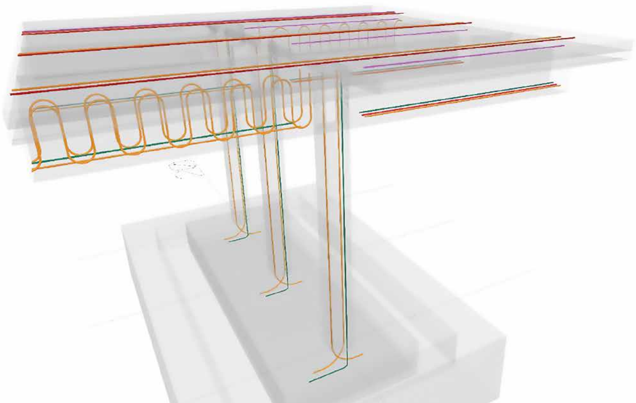
Verteilte faseroptische Sensoren bilden ein künstliches Nervensystem der Brücke (Visualisierung: Hentschke Bau GmbH, Bautzen)
